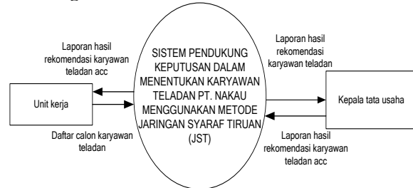
Gambar 5. Diagram Konteks (Context Diagram)
